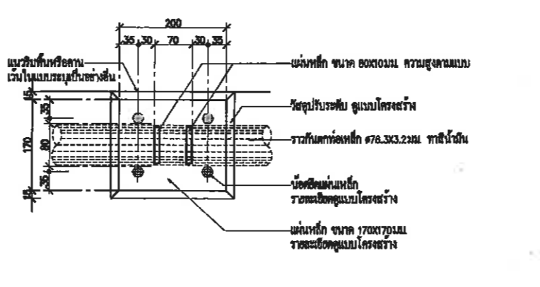
แบบขยายขารับราวบันไดและราวกันตก C5 มาตราส่วน 1: 5 AT A1, 1: 10 AT A3
