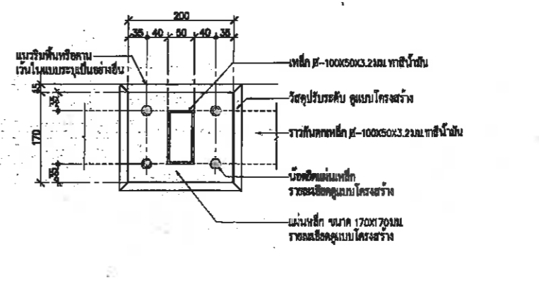
แบบขยายขารับราวบันไดและราวกันตก C3 มาตราส่วน 1: 5 AT A1, 1: 10 AT A3
