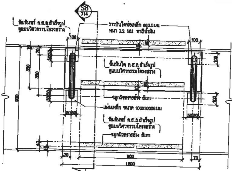
แบบขยายบันไดทางขึ้นอัตโนมัติ มาตราส่วน 1: 10 AT A1, 1: 20 AT A3
