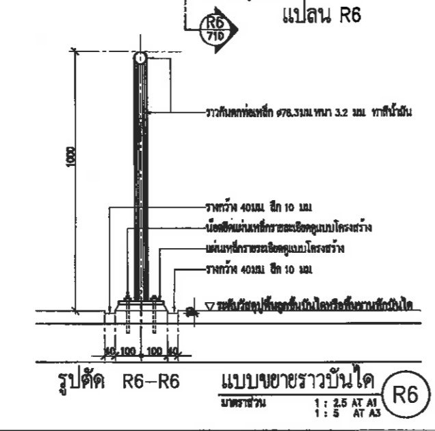
รูปตัด R6-R6 แบบขยายราวบันได (R6) 1: 2.5 AT A1 1: 5 AT A3
