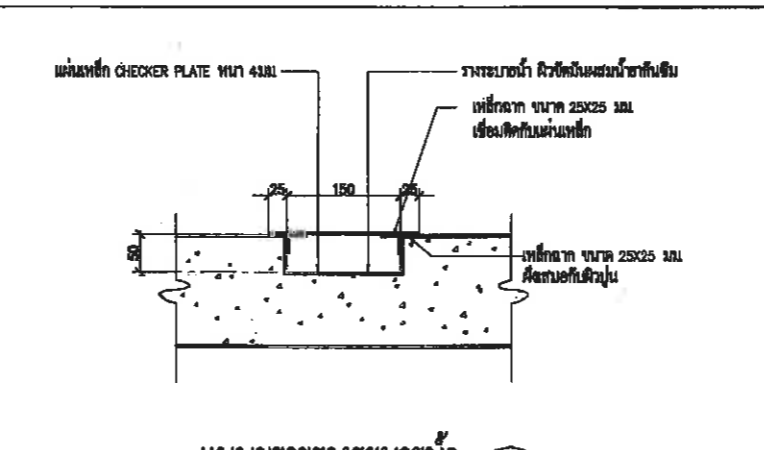
แบบขยายรางระบายน้ำ G2 มาตราส่วน 1: 5 AT A1, 1: 10 AT A3
