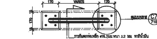
รูปตัด R2-R2 แบบขยายราวบันได (R2) 1: 10 AT A1 1: 20 AT A3
