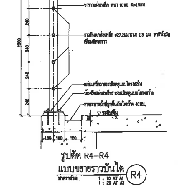
รูปตัด R4-R4 แบบขยายราวบันได (R4) 1: 10 AT A1 1: 20 AT A3
