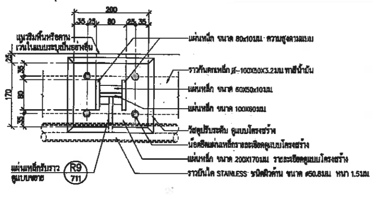
แบบขยายขารับราวบันไดและราวกันตก C1 มาตราส่วน 1: 5 AT A1, 1: 10 AT A3
