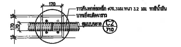
รูปตัด R1-R1 แบบขยายราวบันได (R1) 1: 10 AT A1 1: 20 AT A3
