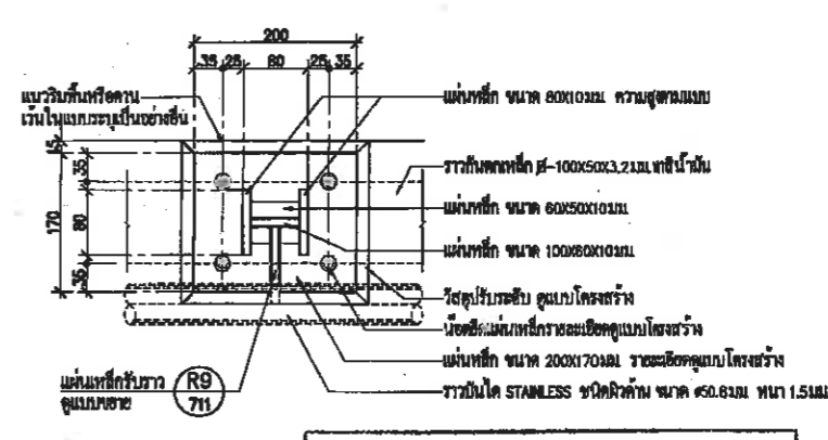
แบบขยายขารับราวบันไดและราวกันตก C6 มาตราส่วน 1: 5 AT A1, 1: 10 AT A3
