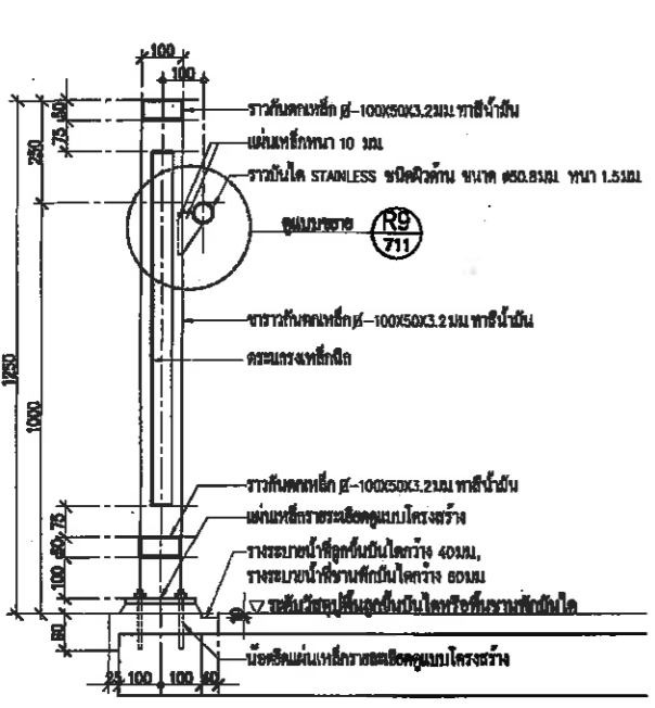
รูปตัด R1-R1 แบบขยายราวบันได (R1) 1: 10 AT A1 1: 20 AT A3
