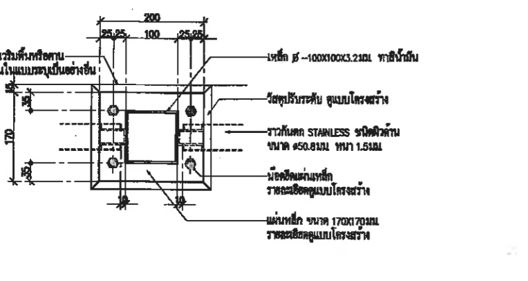
แบบขยายขารับราวบันไดและราวกันตก C4 มาตราส่วน 1: 5 AT A1, 1: 10 AT A3
