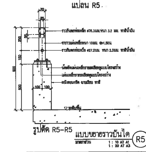
รูปตัด R5-R5 แบบขยายราวบันได (R5) 1: 10 AT A1 1: 20 AT A3
