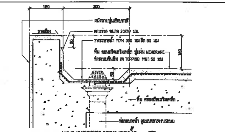
แบบขยายรางระบายน้ำ G3 มาตราส่วน 1: 5 AT A1, 1: 10 AT A3
