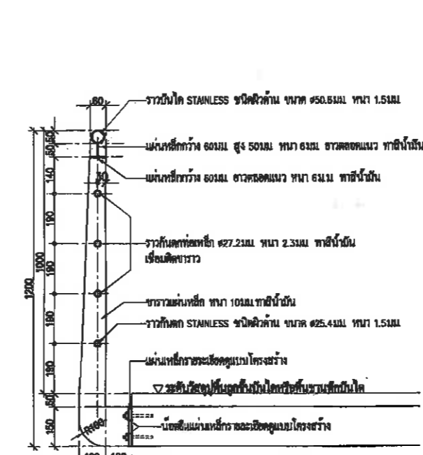
รูปตัด R3-R3 แบบขยายราวบันได (R3) 1: 10 AT A1 1: 20 AT A3
