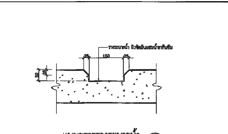
แบบขยายรางระบายน้ำ G1 มาตราส่วน 1: 5 AT A1, 1: 10 AT A3
