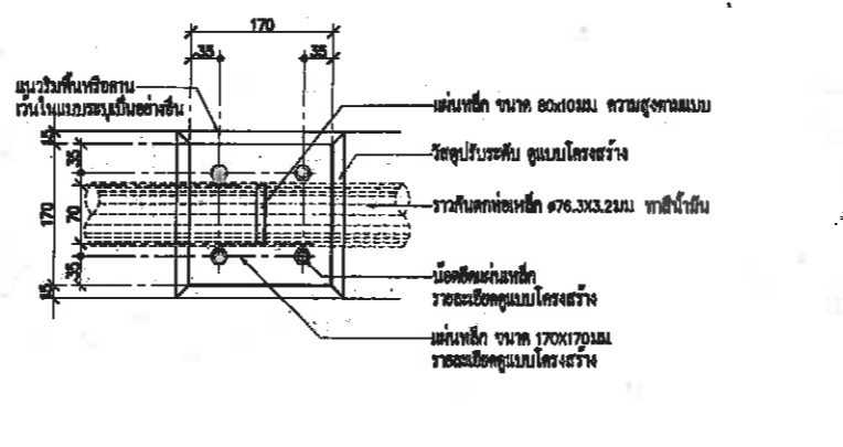
แบบขยายขารับราวบันไดและราวกันตก C2 มาตราส่วน 1: 5 AT A1, 1: 10 AT A3
