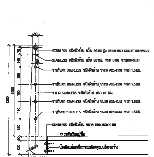
รูปตัด R2-R2 แบบขยายราวบันได (R2) 1: 10 AT A1 1: 20 AT A3
