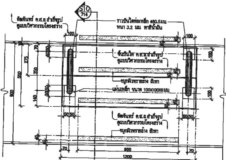
แบบขยายบันไดทางขึ้นอัตโนมัติ มาตราส่วน 1: 10 AT A1, 1: 20 AT A3
